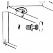
Рис.3 Схема сборки на эксцентриковую стяжку
