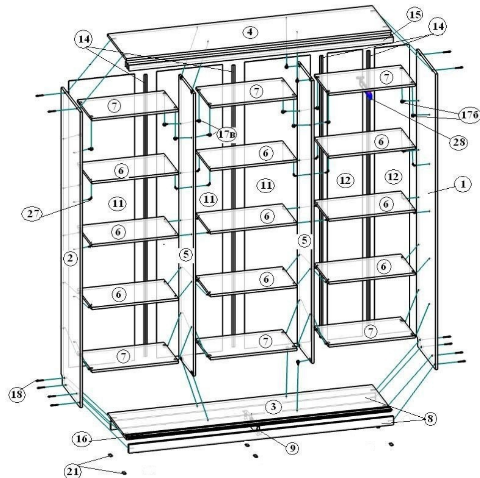
Рисунок 1 Схема сборки библиотеки-купе
