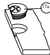
Рис.2 Схема установки эксцентрика
