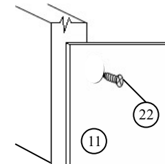
Рис.4 Схема крепления задней стенки к корпусу
